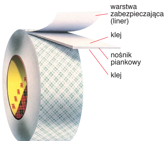
Tymczasowe mocowanie plakatów reklamowych (taśma 4658F)
